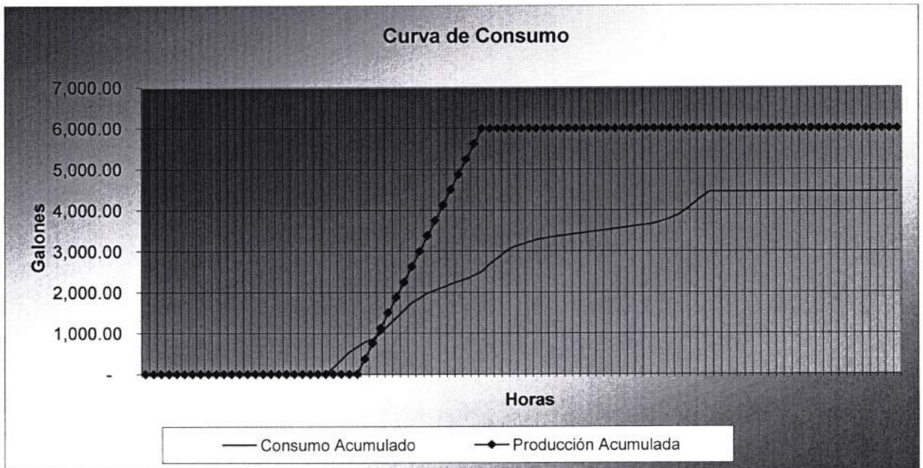
Ilustración 1. Distribución de consumo de agua en las horas de uso estimado.
