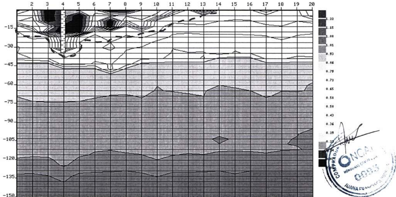
Figura 3. Perfil de Potencial Natural #1.
