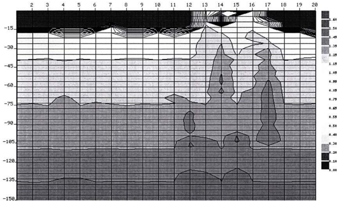
Figura 5. Perfil de Potencial Natural #2.
